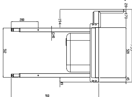
Zij aanzicht
