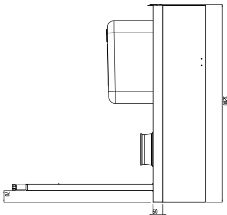
Zij aanzicht
